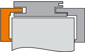
Переріз дверної коробки
