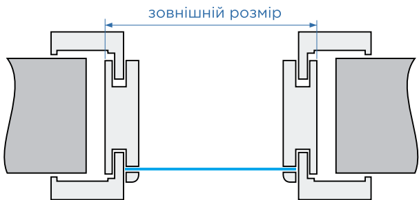
Конструкція фрамуги у виконанні Verto-FIT
