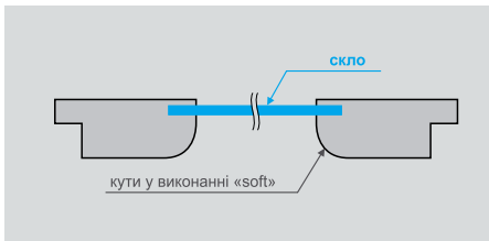
Скло встановлено зі зміщенням під фальц полотна з заокругленими кутами (soft)
