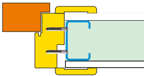
Монтаж в гіпсокартонну стіну за допомогою кріпильних гвинтів
