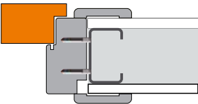
Монтаж в гіпсокартонну стіну за допомогою гвинтів
