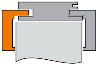
Переріз дверної коробки
