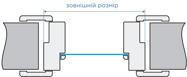
Конструкція фрамуги у виконанні STANDARD
